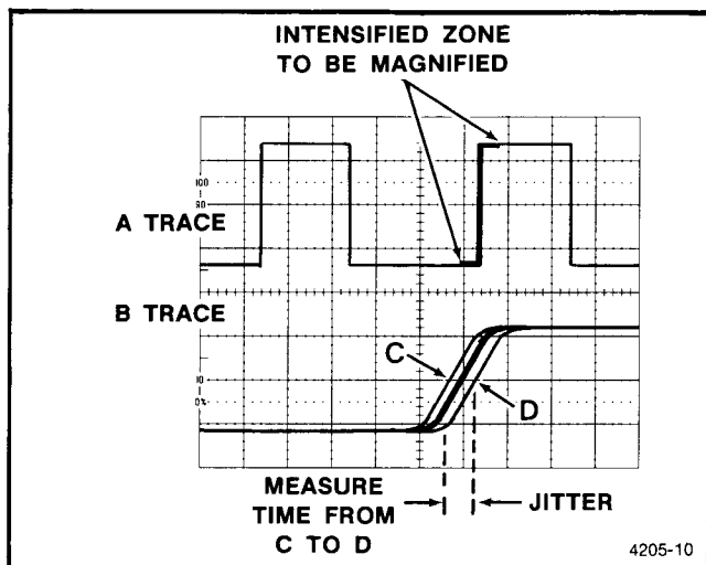
Fig. 4-6. Pulse jitter.
